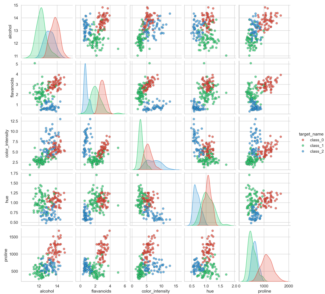
Рисунок 6 — Скаттер-плоты пар признаков с разделением по классам
